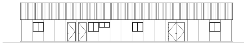
정면도
